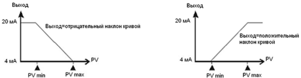
рис. 1 Пропорциональная выходная диаграмма
