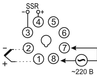
SSR – управление твердотельным реле
