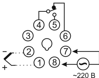
Реле ~5 А, 250 В
