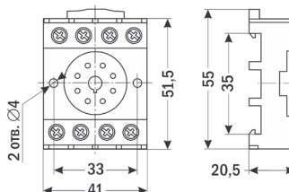
Клеммная колодка
