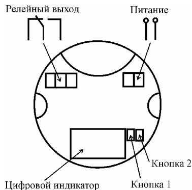
Рис.3 Схема подключения
